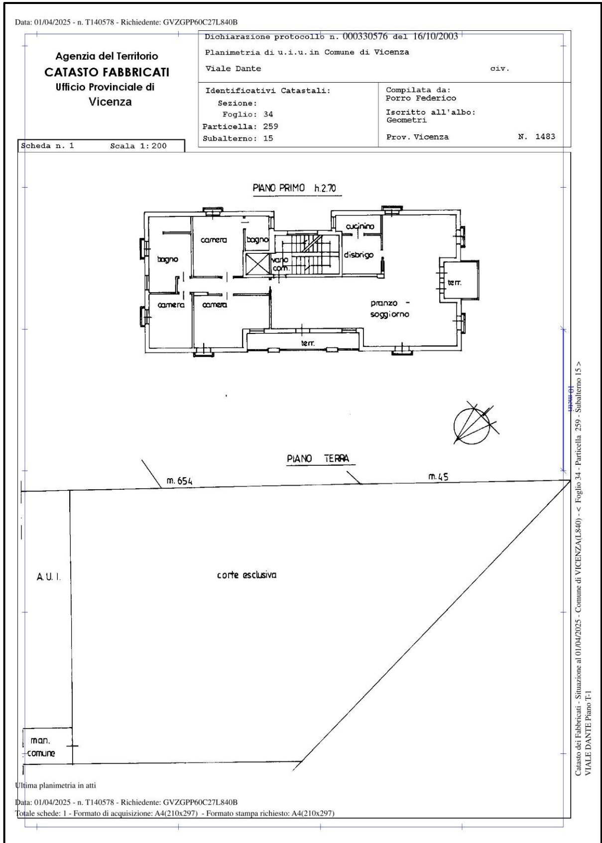
Planimetria subalterno 15
