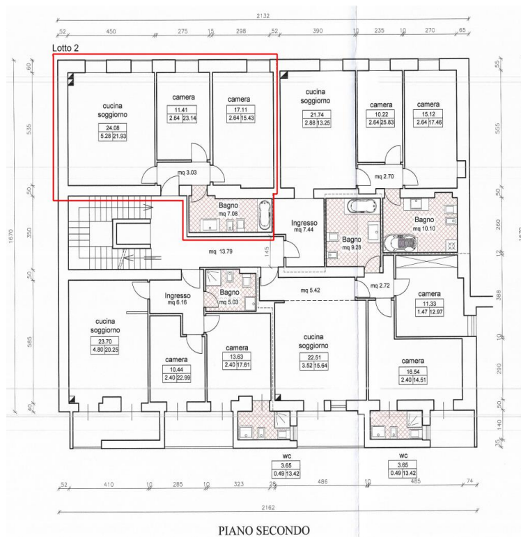
Figura 3. Planimetria immobili (Allegato 6)
