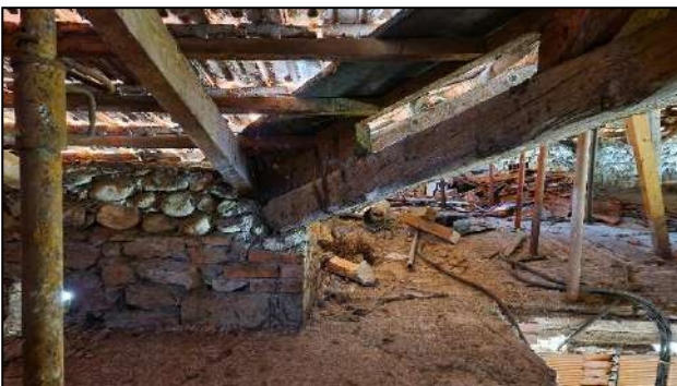
Trave cantonale di compluvio della copertura
