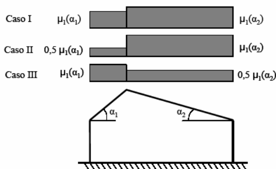
Condizioni di carico per coperture a due falde (Fig. 3.4.3 delle NTC 2018)
