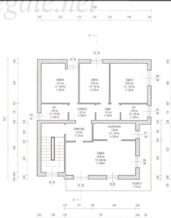
STATO DI PROGETTO PIANO SECONDO DIA IN VARIANTE N. 65/2003 DEL 01.07.2003 ALLA C.E. N. 8/2002;
