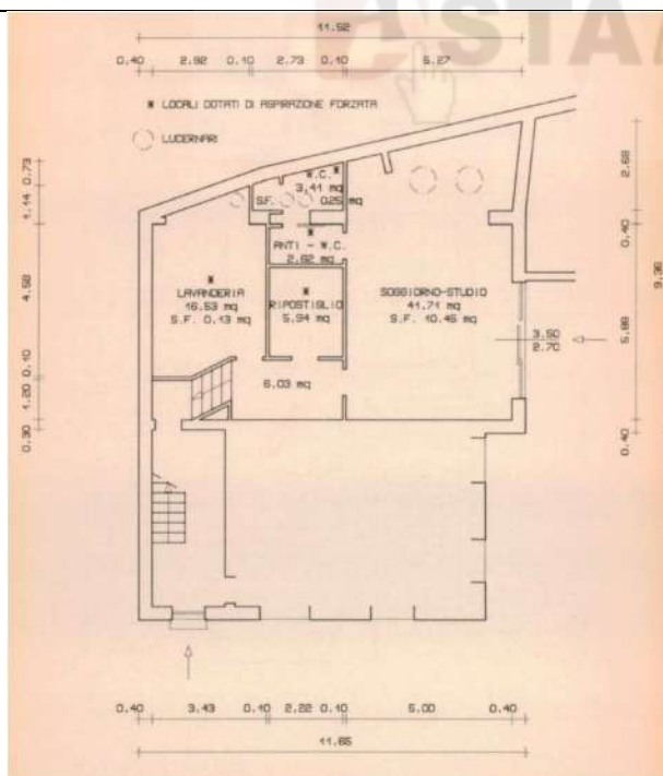
STATO DI PROGETTO PIANO TERRA
