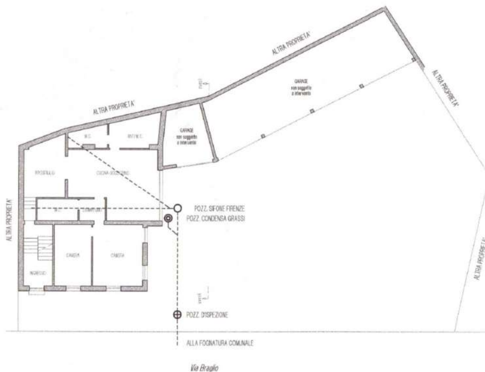
STATO DI PROGETTO PIANO TERRA DIA IN VARIANTE N. 65/2003 DEL 01.07.2003 ALLA C.E. N. 8/2002;
