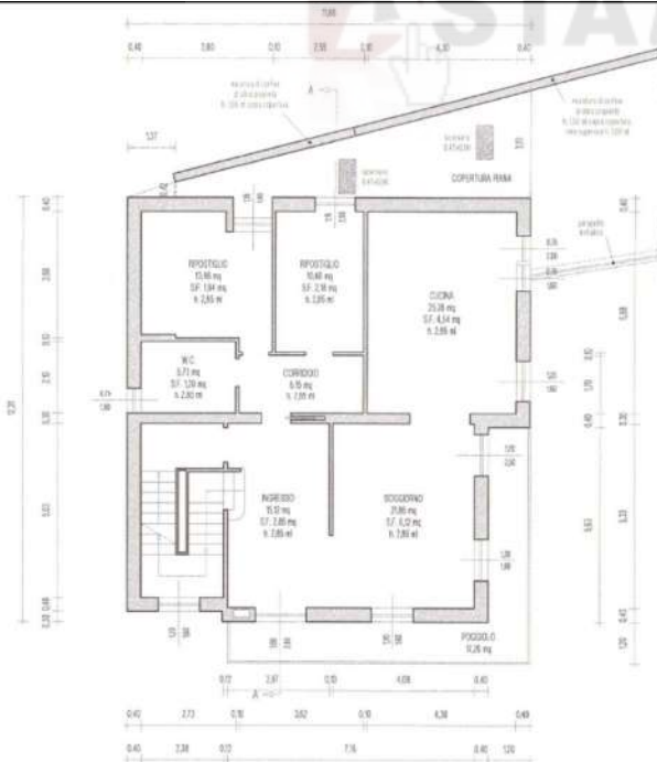
STATO DI PROGETTO PIANO PRIMO DIA IN VARIANTE N. 65/2003 DEL 01.07.2003 ALLA C.E. N. 8/2002;
