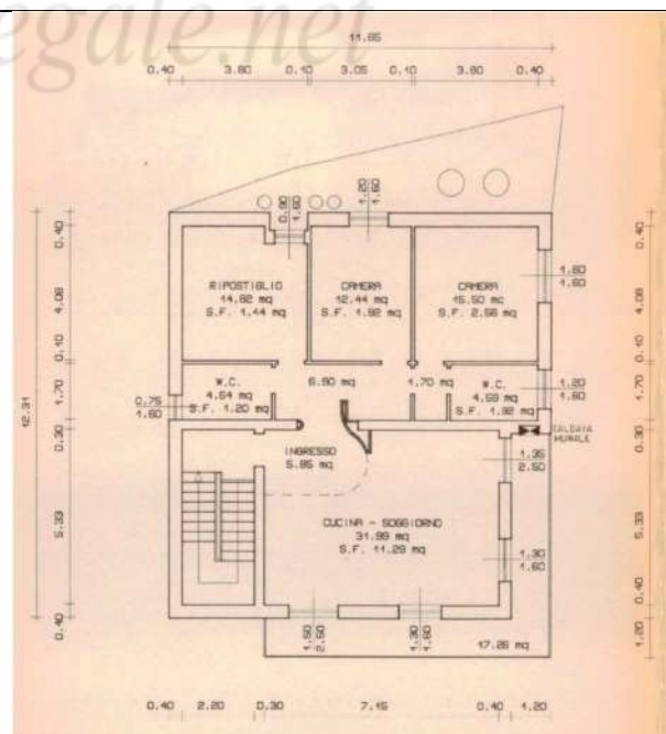
STATO DI PROGETTO PIANO SECONDO
