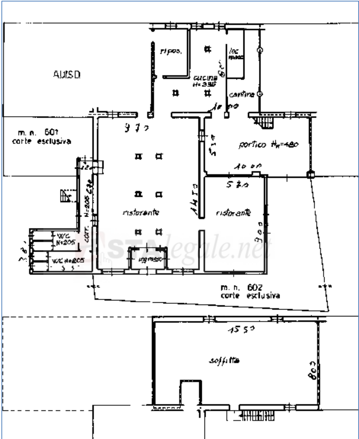
Edificio Fig. 15 Particella 393 Sub 3 - Pianta piano terra e piano primo - stato catastale
