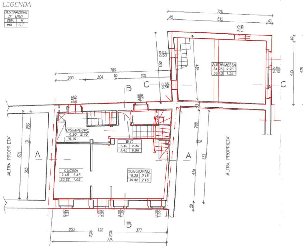
Figura 42. Comparazione stato attuale – stato approvato – piano terra.
