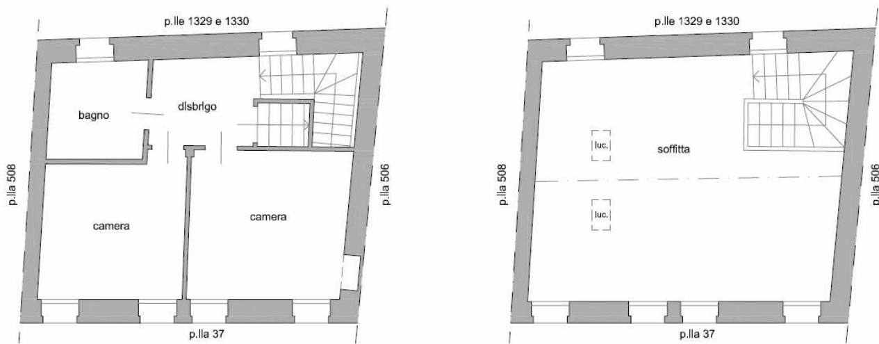
Figura 4. Planimetria piani primo e secondo, p.la 507.
