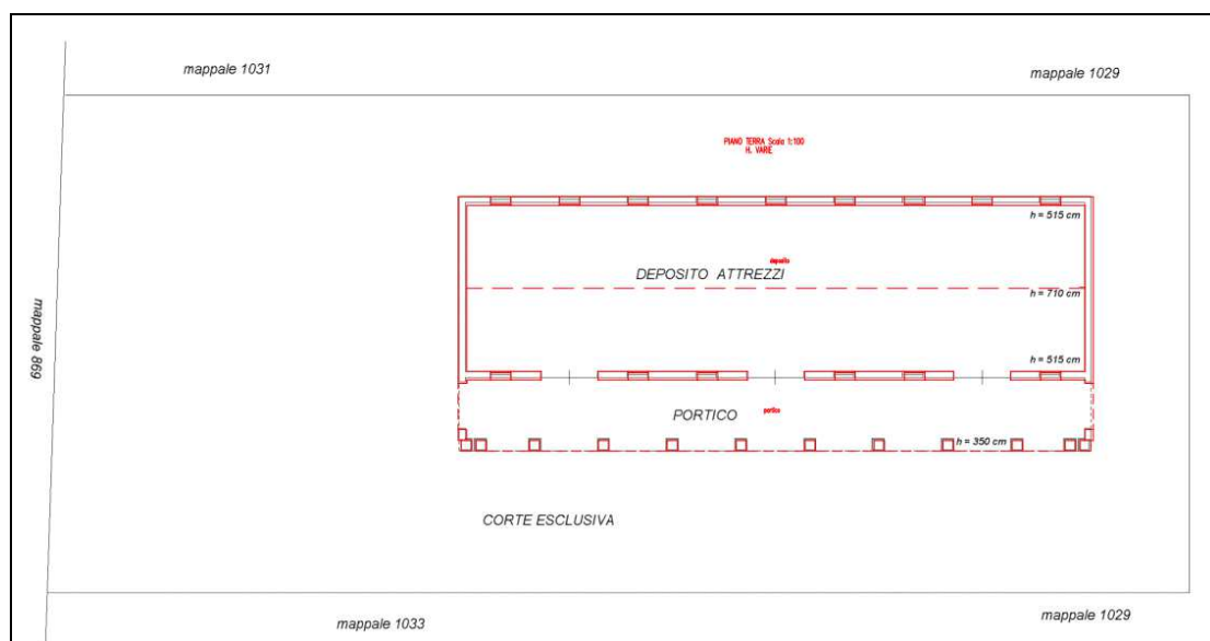
Sovrapposizione rilievo (in rosso) e planimetria catastale (in nero) m.n. 1034 (fuori scala)
