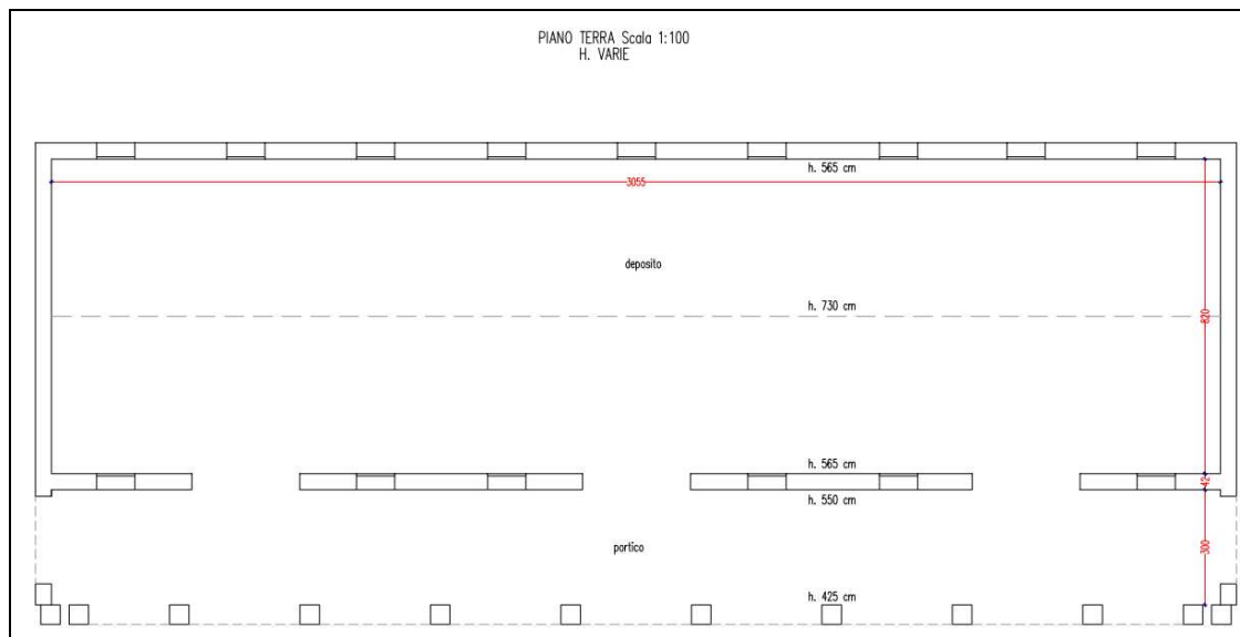
m.n. 1034 piano terra (fuori scala)
