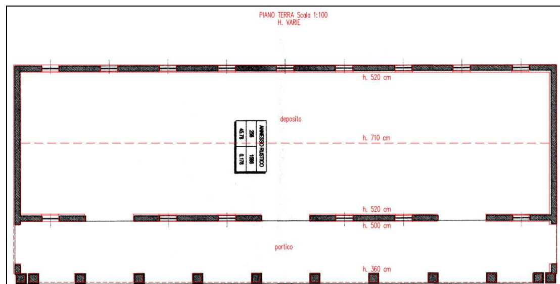
Sovrapposizione rilievo (in rosso) e stato autorizzato (in nero) m.n. 1034 (fuori scala)
