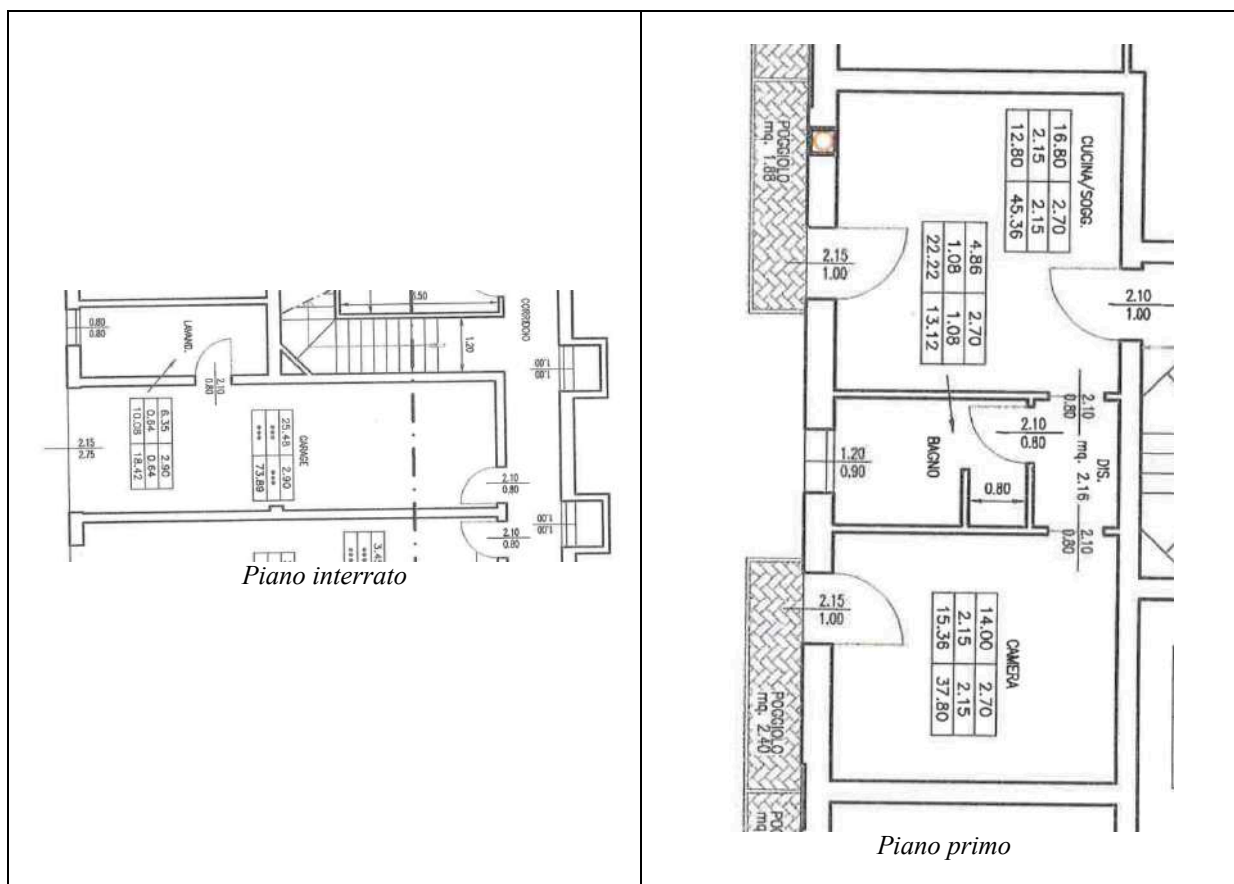
Estratto progetto approvato (non in scala).
