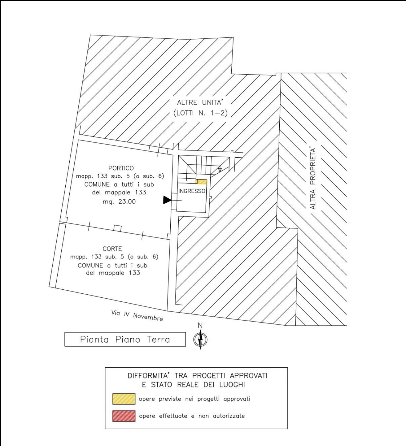
Figura 9.a. Comparazione stato attuale – stato rilevato. Unità mappale 133 sub. 4 / 137 sub. 8 – piano Terra
