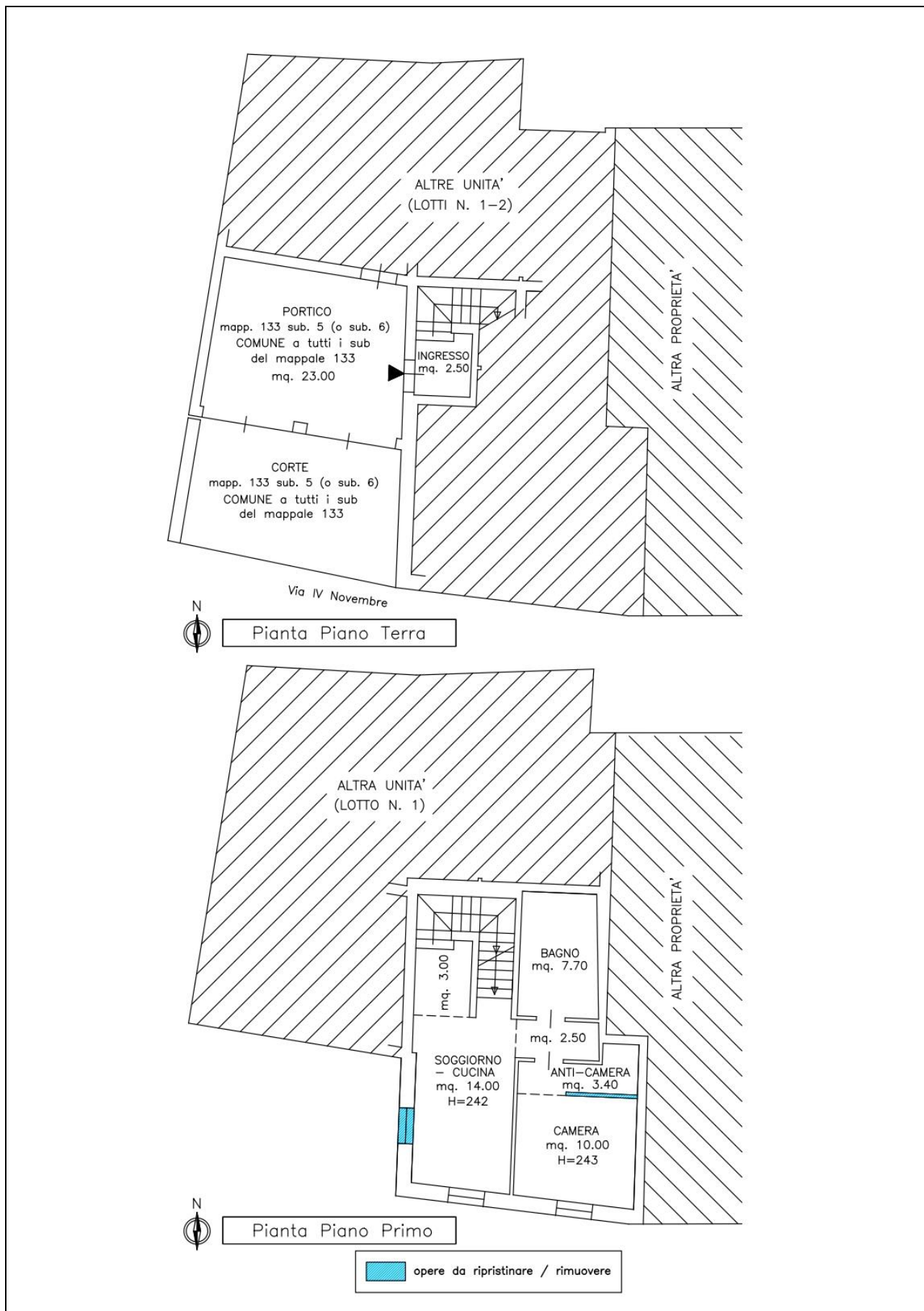
Figura 3.a. Planimetrie immobili – Appartamento mapp. 133 sub. 4 / 137 sub. 8 – Piani Terra e Primo.
