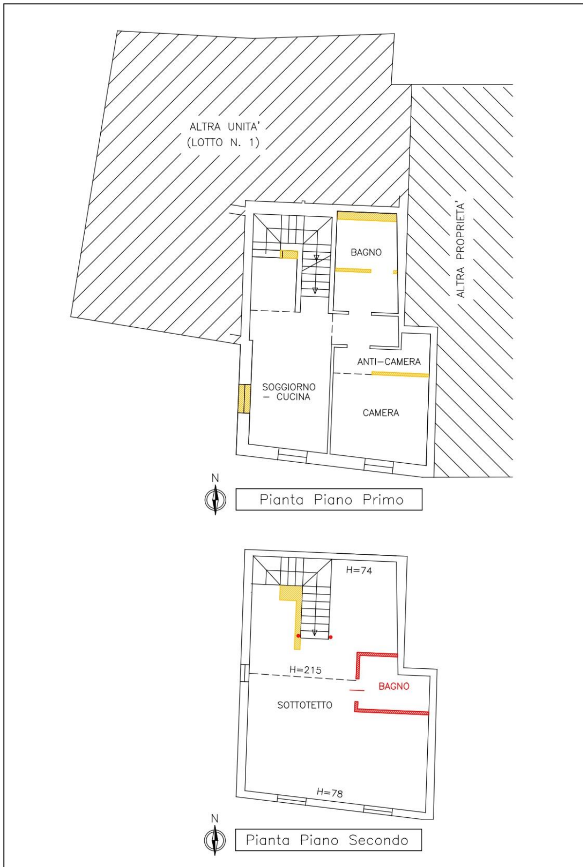
Figura 9.b. Comparazione stato attuale – stato rilevato. Unità mappale 133 sub. 4 / 137 sub. 8 – piani Primo e Secondo
