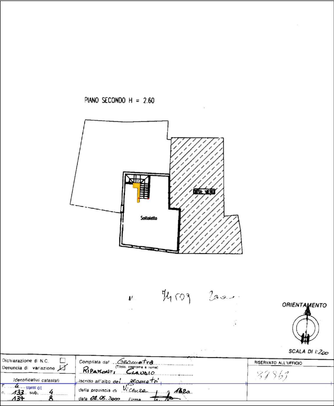
Figura 7.b. Sovrapposizione tra lo stato dei luoghi e la planimetria catastale unità mappale 133 sub. 4 / 137 sub. 8 – piano Secondo
