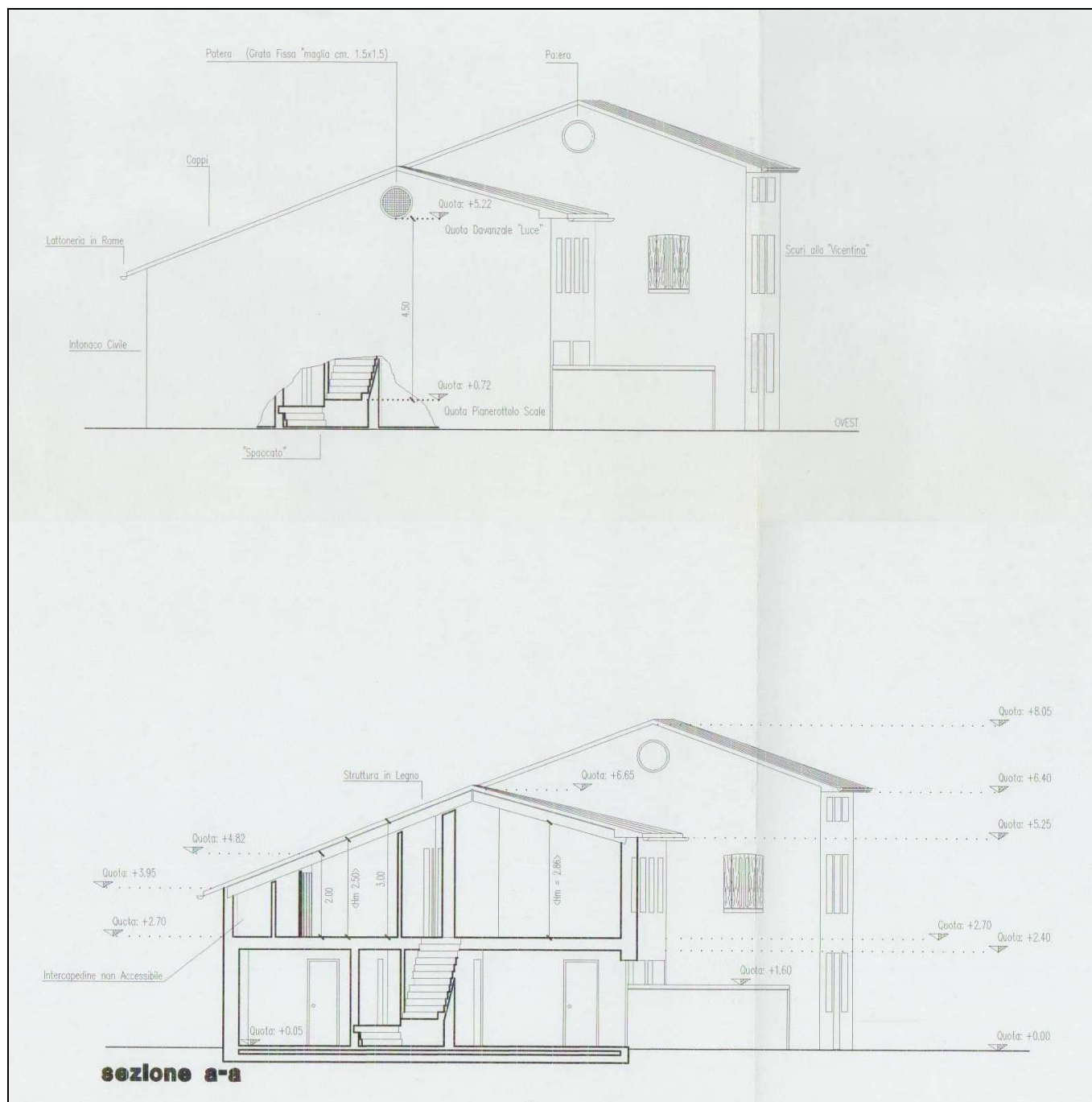
Figura 10.d. Stato approvato: unità mappale 133 sub. 4 / 137 sub. 8 - Prospetto Ovest – Sezione a-a (Comunicazione di Inizio attività in data 11.04.2000 prot. 4012).
