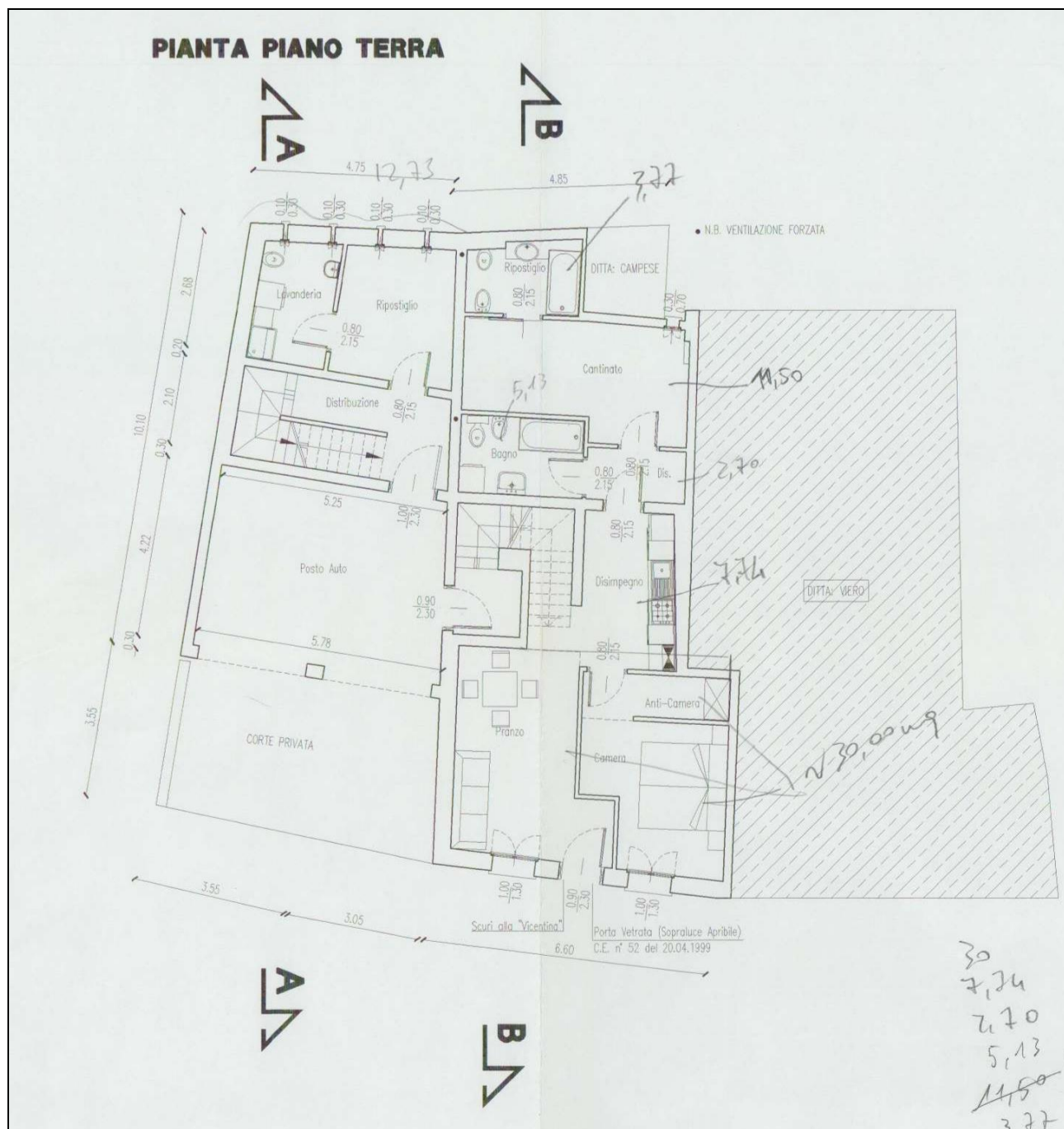
Figura 10.a. Stato approvato: unità mappale 133 sub. 4 / 137 sub. 8 - Pianta Piano Terra (Comunicazione di Inizio attività in data 11.04.2000 prot. 4012).
