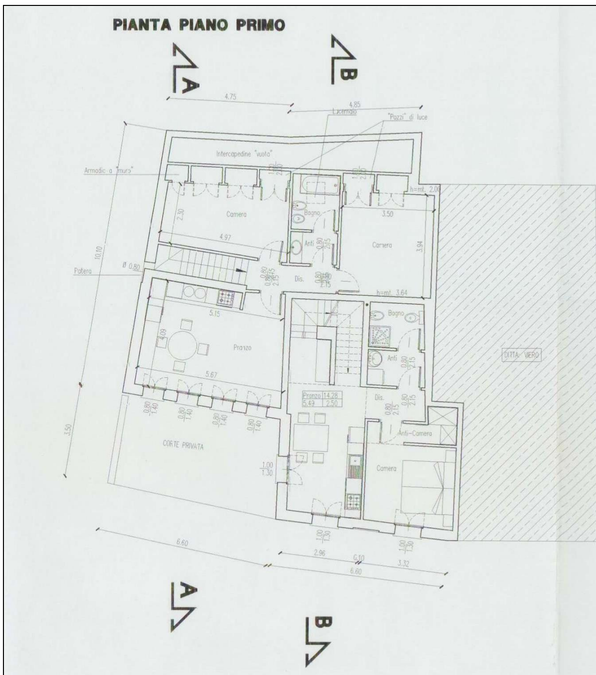
Figura 10.b. Stato approvato: unità mappale 133 sub. 4 / 137 sub. 8 - Pianta Piano Primo (Comunicazione di Inizio attività in data 11.04.2000 prot. 4012).
