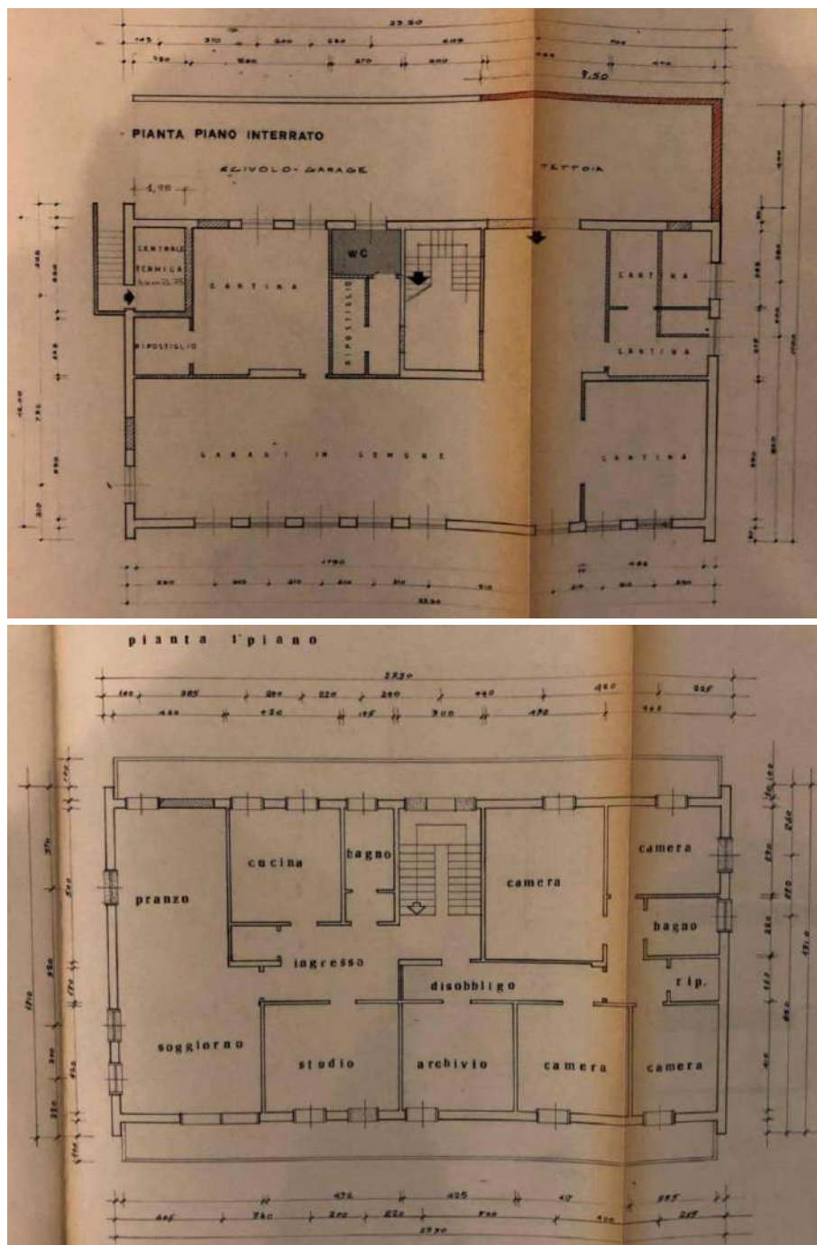
Figura 9. Stato approvato.
