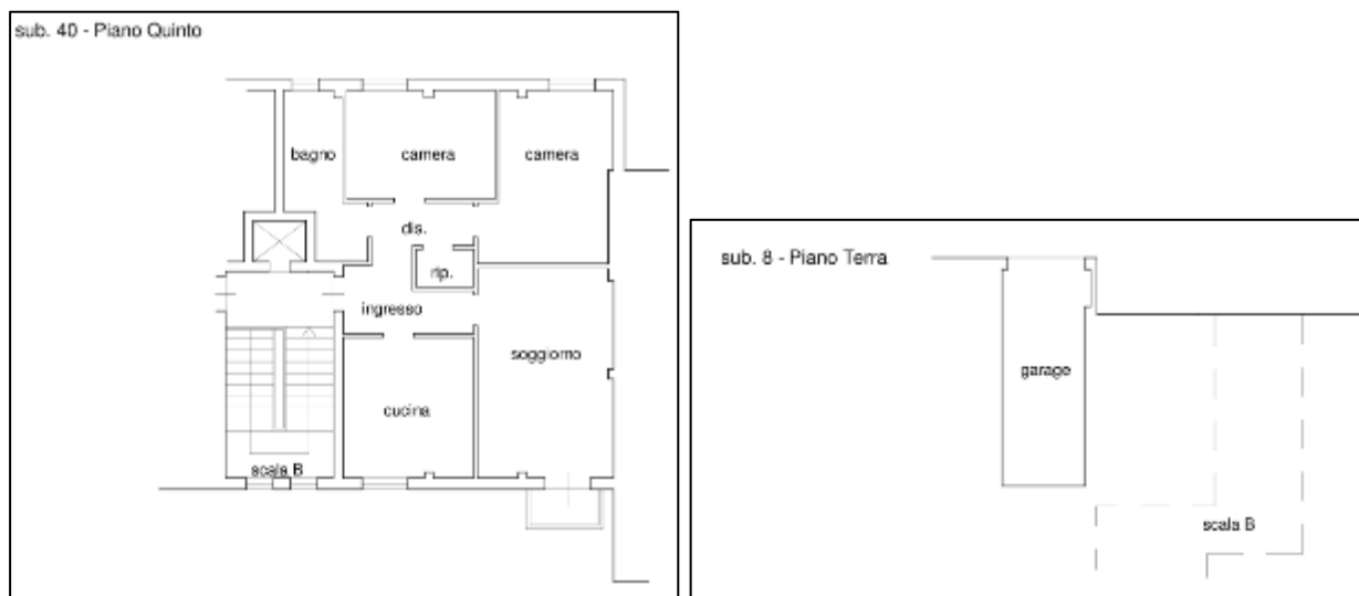
Figura 3. Schema planimetrico stato dei luoghi
