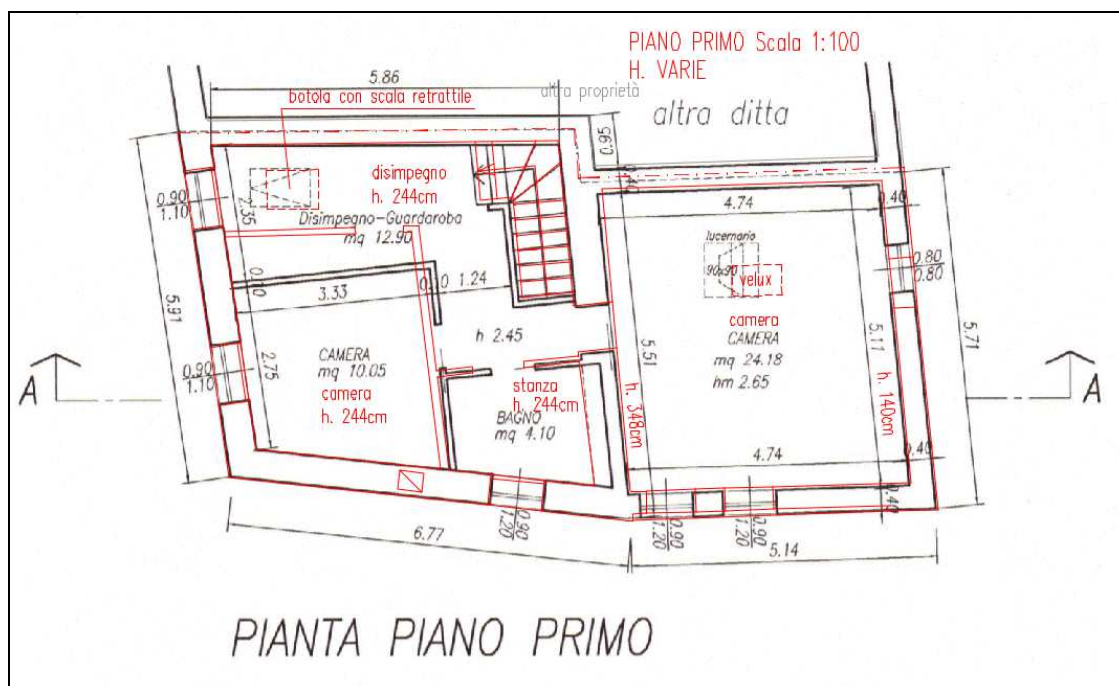
Comparazione stato autorizzato – stato rilevato - piano primo
