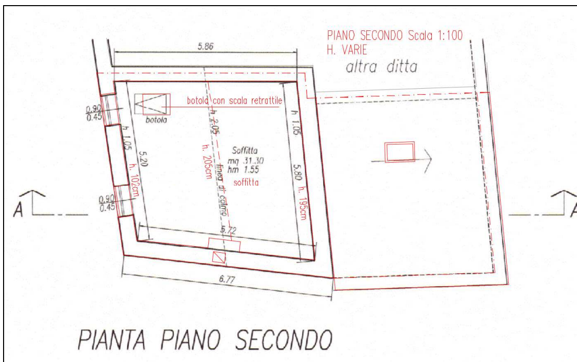
Comparazione stato autorizzato – stato rilevato – secondo
