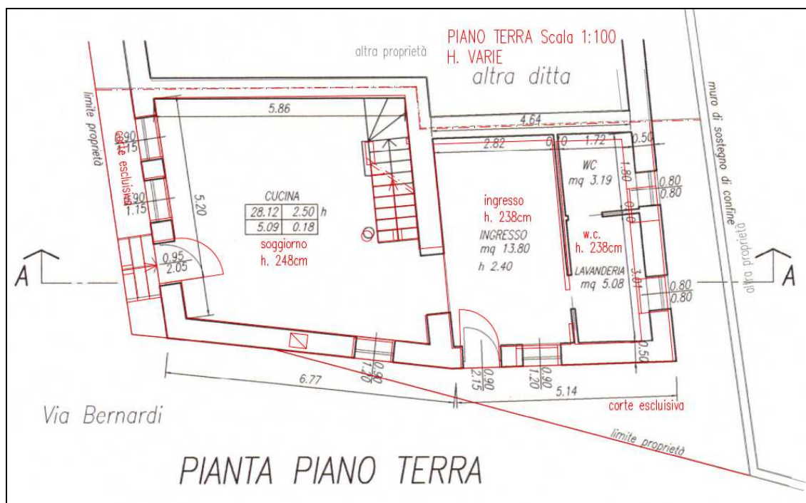
Comparazione stato autorizzato – stato rilevato - piano terra
