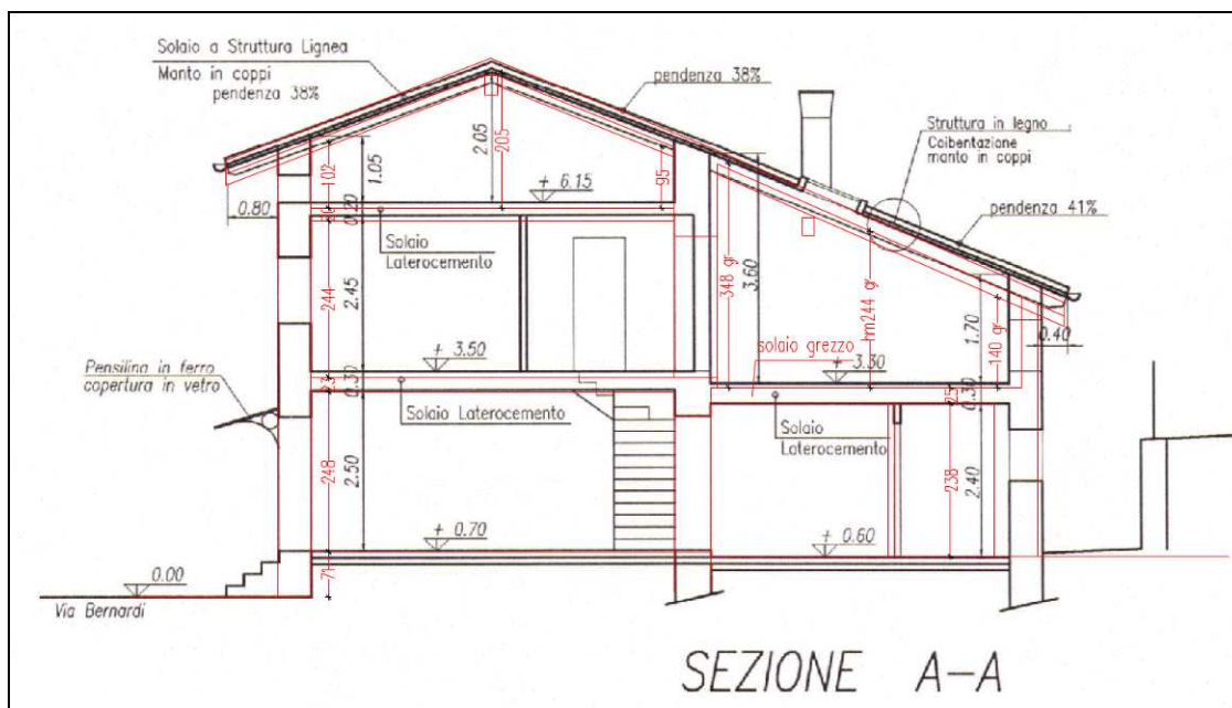
Comparazione stato autorizzato – stato rilevato - sezione
